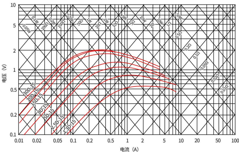
XXD-15电压-电流曲线
